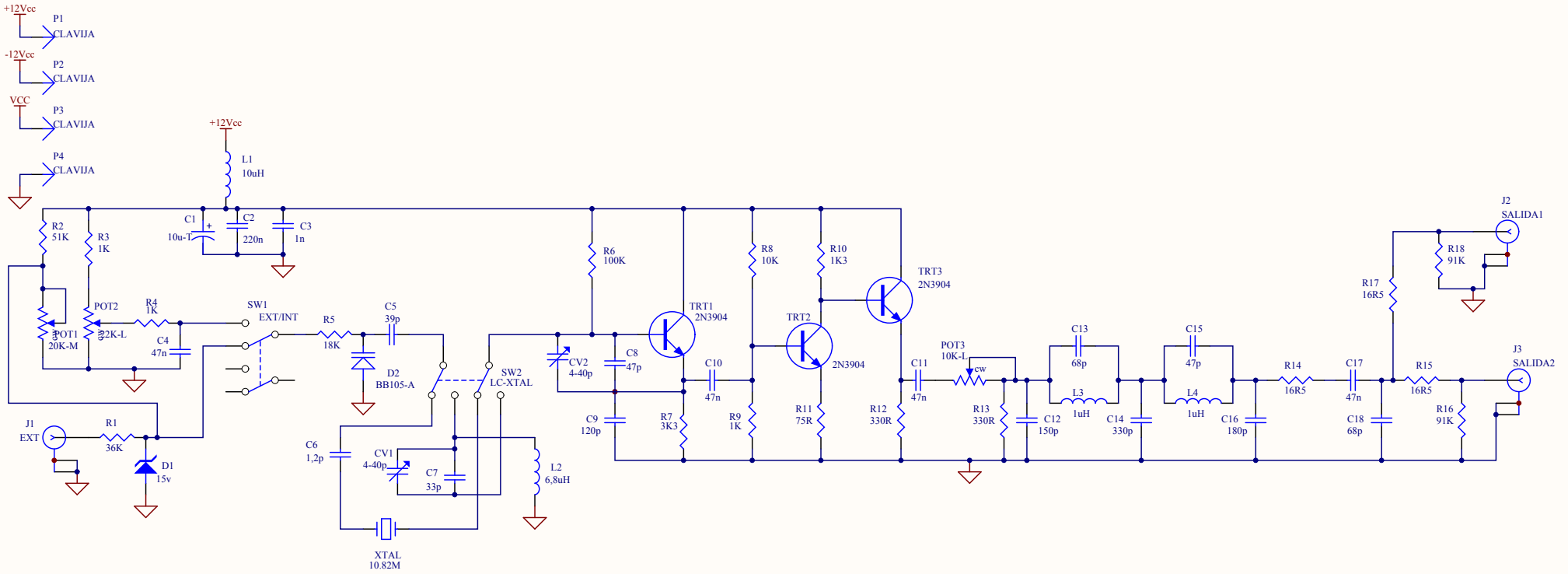
OSCILADOR LOCAL FI (10.82MHz)
